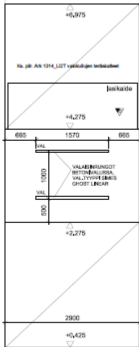
PROJEKTIO C 1/25
